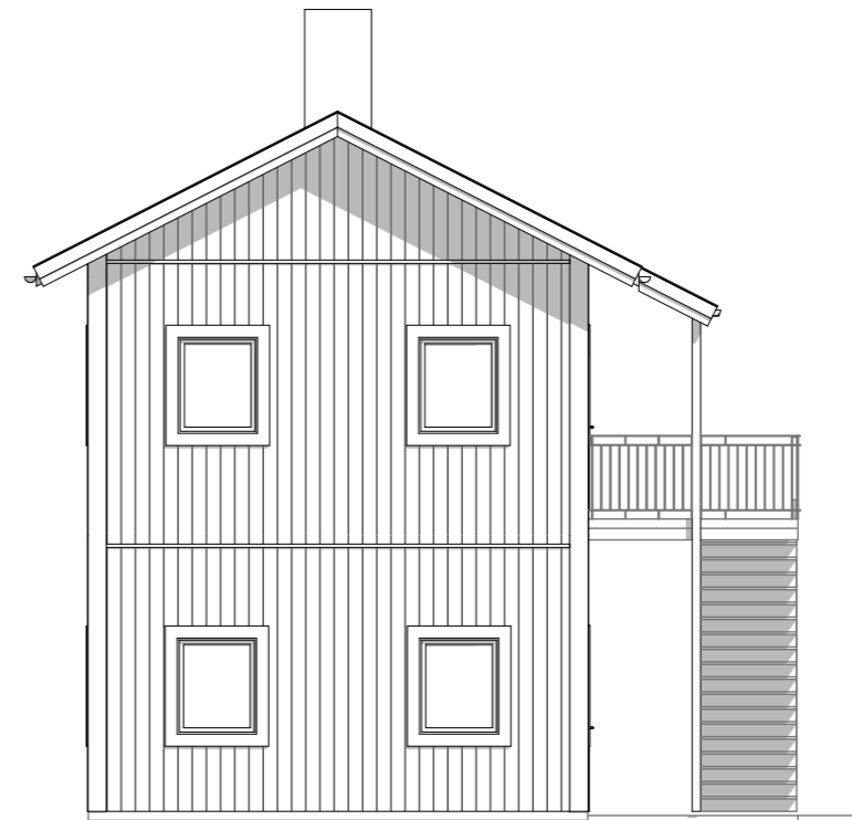
F7 Fasad 1:100
