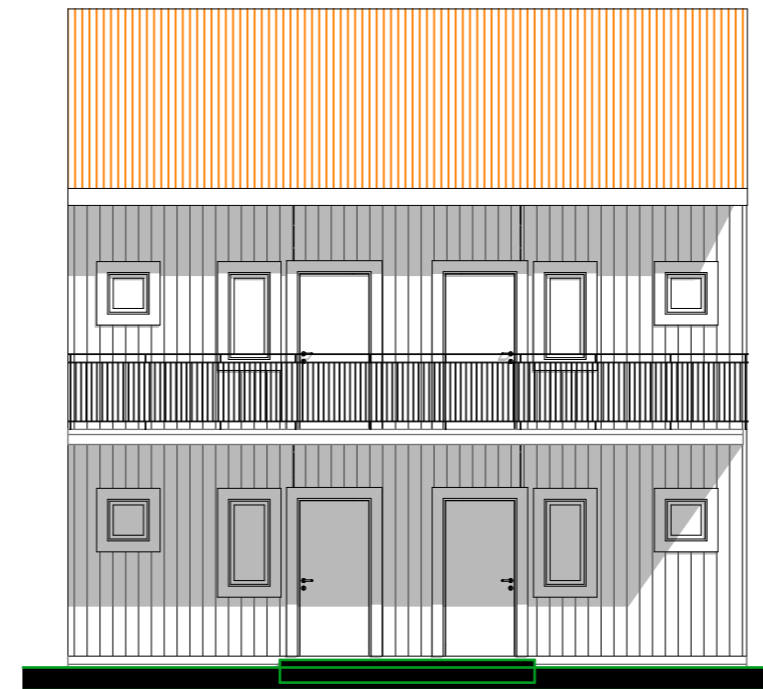
F9 Fasad 1:100
